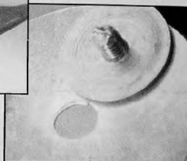
Крепление в сборе. Видна накатка на гурте вертнего болта для удобства отворачивания.
